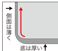
スピニング加工による軽量化
